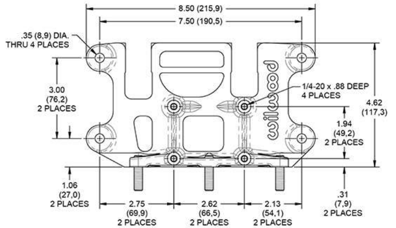
VIEW A-A
